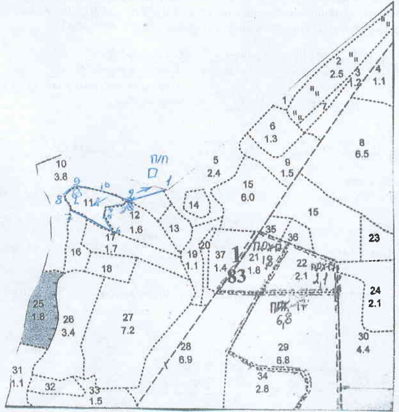
Абрис лесосеки с указанием основных элементов (технологические полосы, волокна, технологические (погрузочные) пункты)
