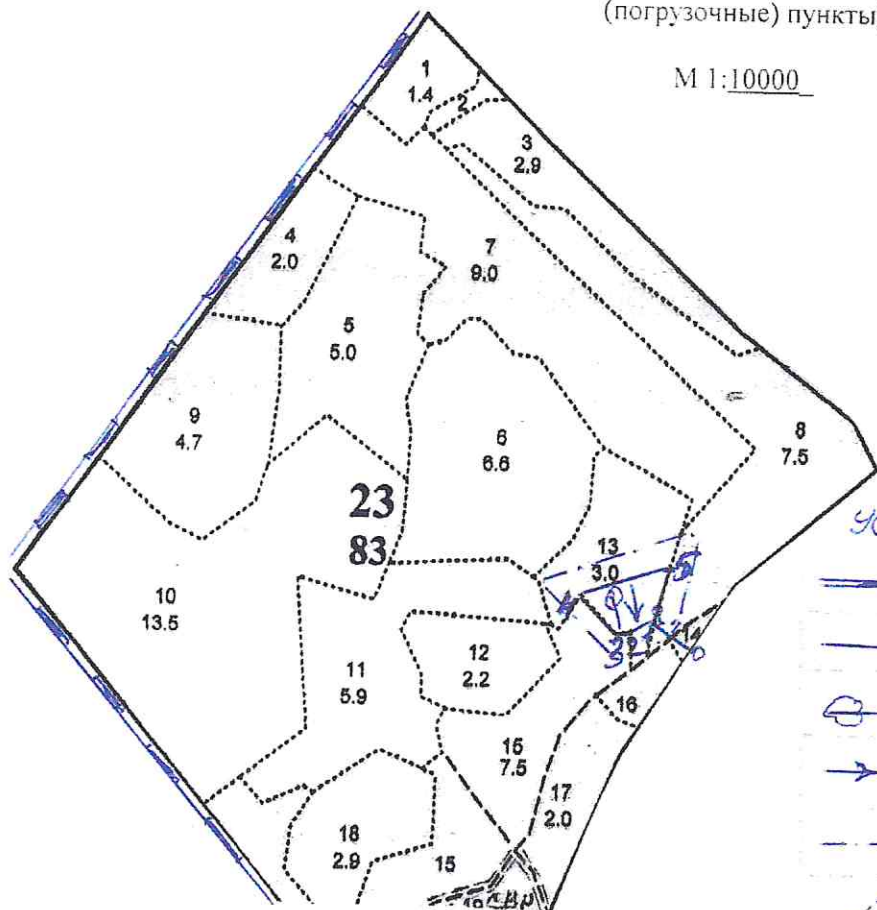
Абрис лесосеки с указанием основных элементов (технологические полосы, валки, технологические (погрузочные) пункты)
