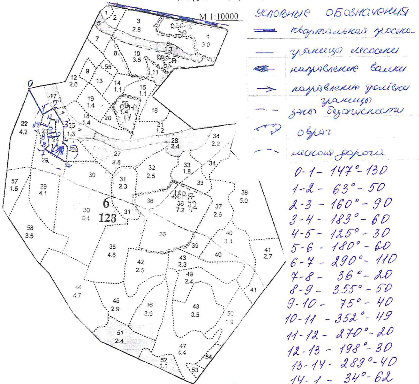
Абрис лесосеки с указанием основных элементов (технологические полосы, волоки, технологические (погрузочные) пункты)
