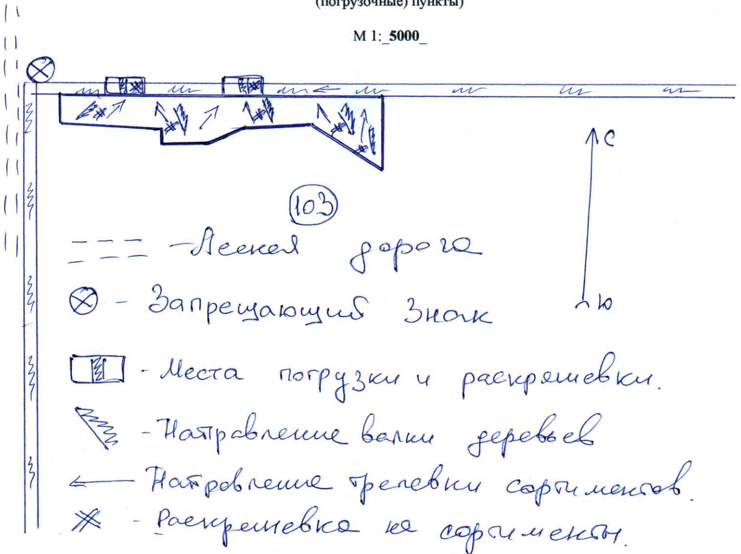
Абрис лесосеки с указанием основных элементов (технологические полосы, волоки, технологические (погрузочные) пункты)
